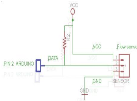
GAMBAR 3. Rangkaian Skematik Sensor Flow Meter
