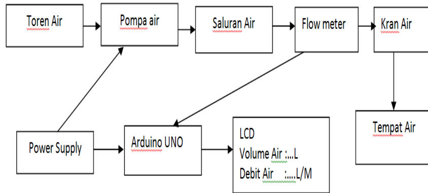
GAMBAR 2. Blok Alur Pengukuran Digital Meter Air
