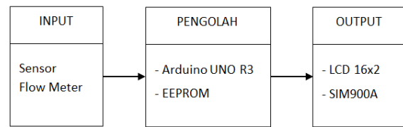
Gbr. 2 Diagram Proses Pembacaan Volume dan Debit Air
