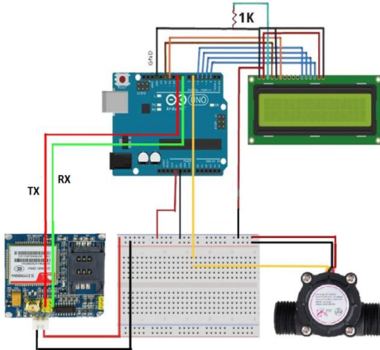
Gbr. 1 Diagram Rangkaian Alat Pencatatan Meter Air Digital
