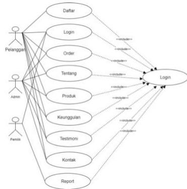
Gambar 4. Use Case Diagram Pemesanan
