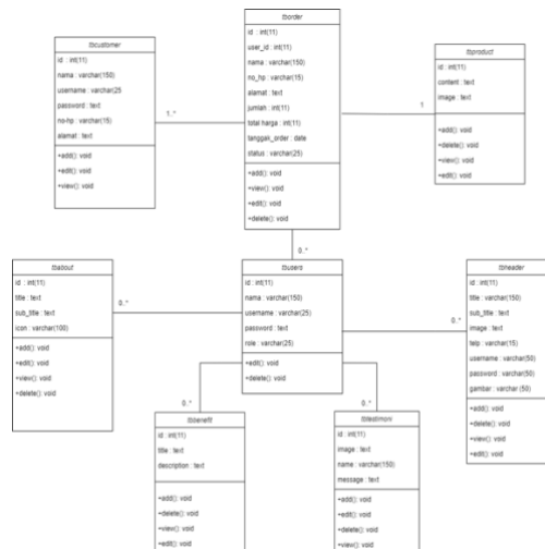
Gambar 7. Class Diagram Pemesanan
